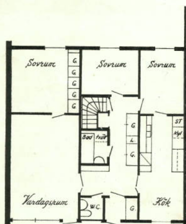
överplan
