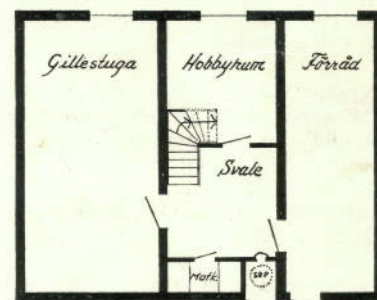
källarplan
