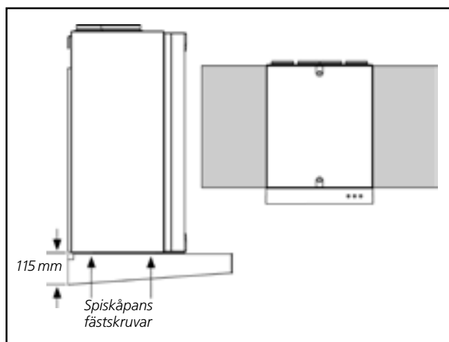
El- och styrkablar samt anslutningen för spiskåpans frånluft finns under täckplattorna i aggregatets botten.
